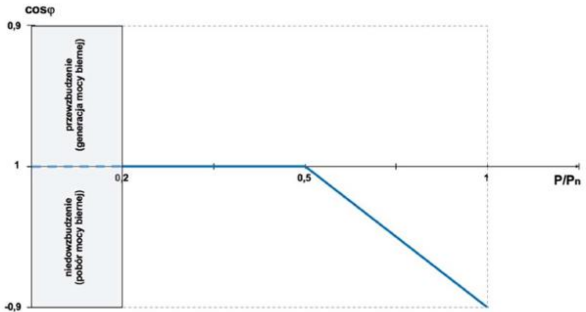
Rys. 5 Charakterystyka sterowania współczynnikiem mocy \cos \varphi w funkcji generowanej mocy czynnej wymagana przez OSD.
